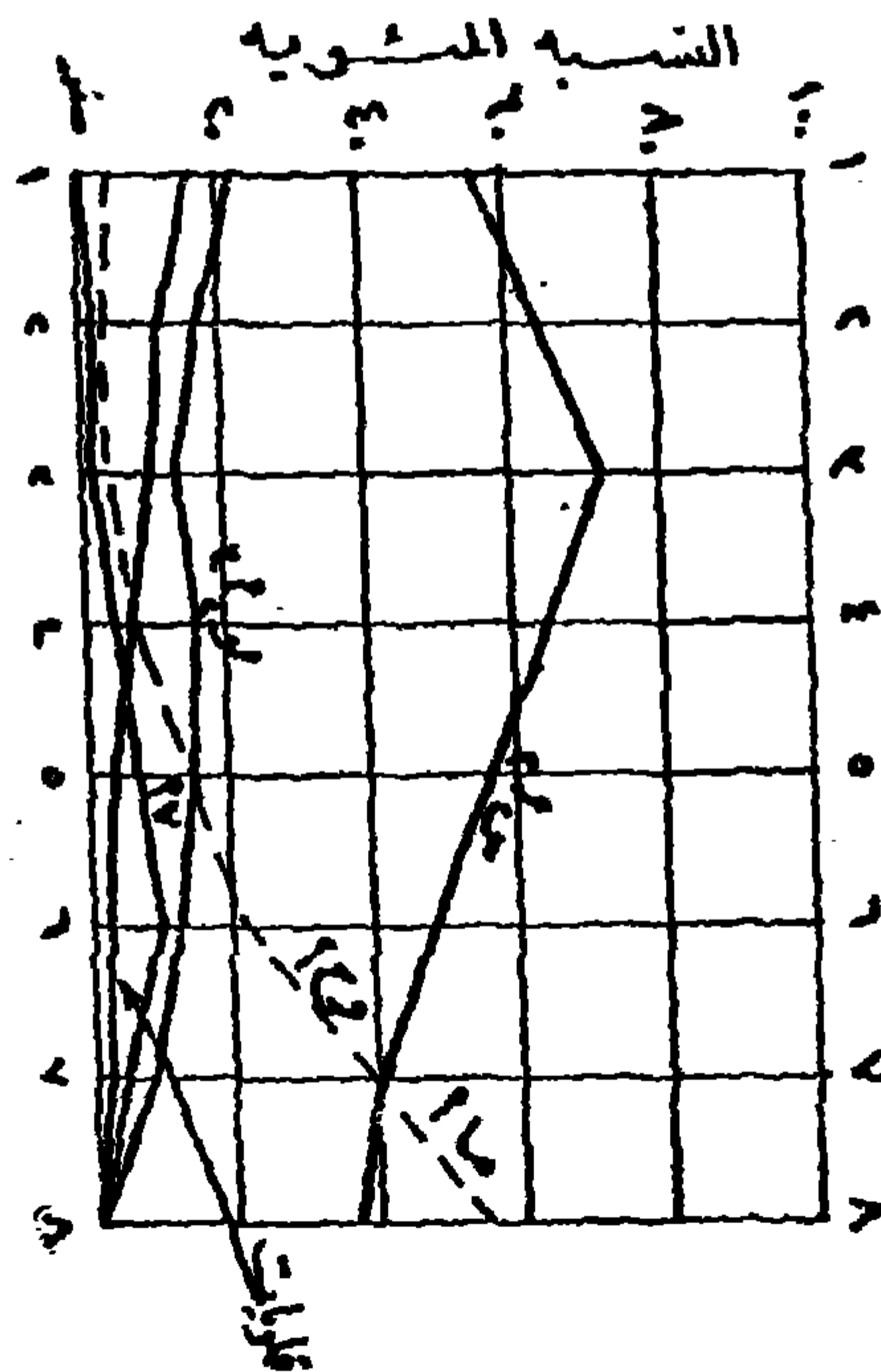
( شكل رقم ٢ ) « التركيب الكيميائي العام للصخور النارية العادية »
